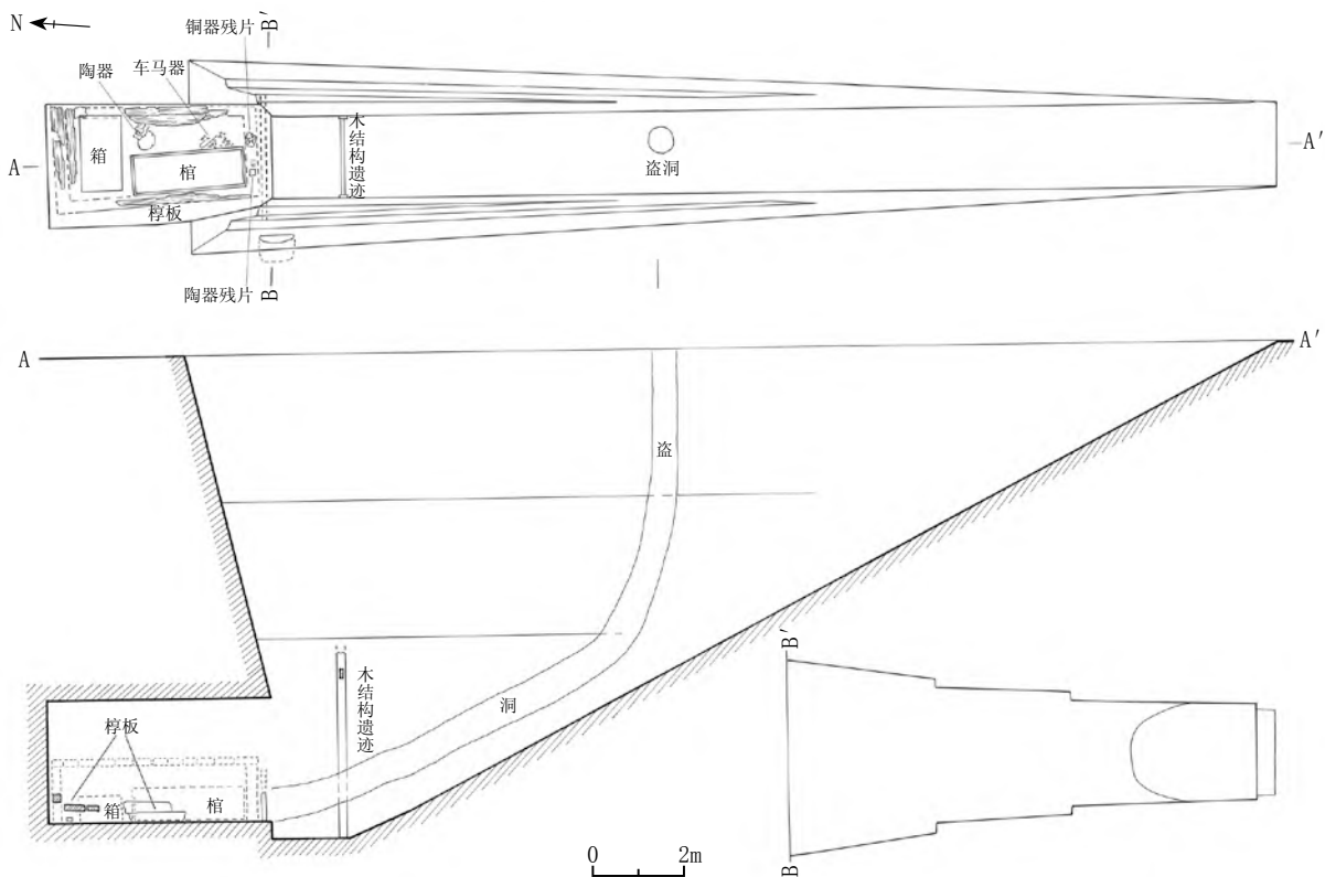
图四 97GYM130 平面、剖视图及洞室口剖面图
